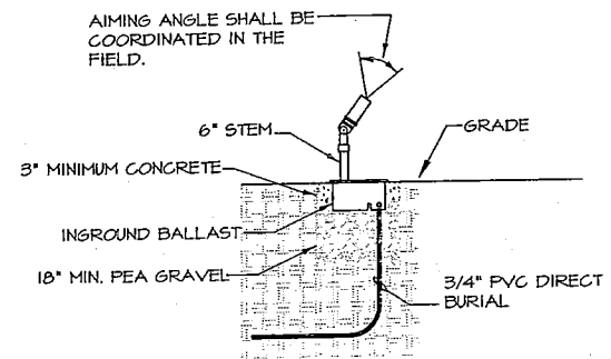
FIXTURE SA & SB BASE DETAIL NO SCALE
