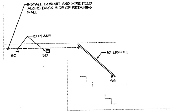
STAIR ELEVATION B SCALE: 1/4" = 1'-0"
